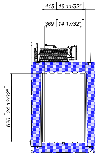
Sezione F-F
