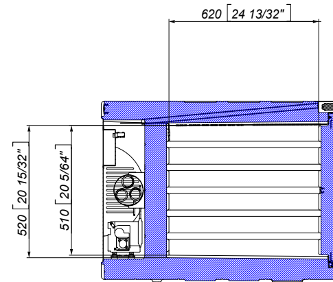
Sezione E-E
